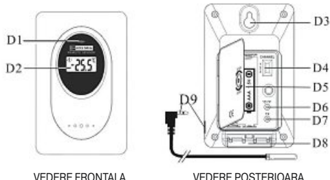
VEDERE FRONTALA
