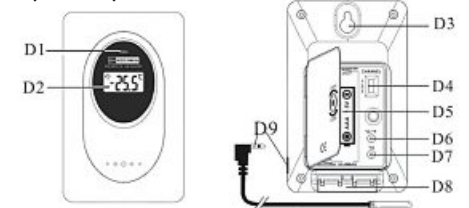
Фронтален изглед
