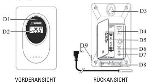
VORDERANSICHT
